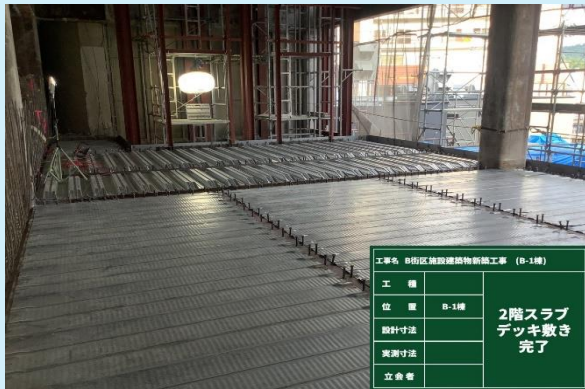
2階 デッキ敷込完了状況
